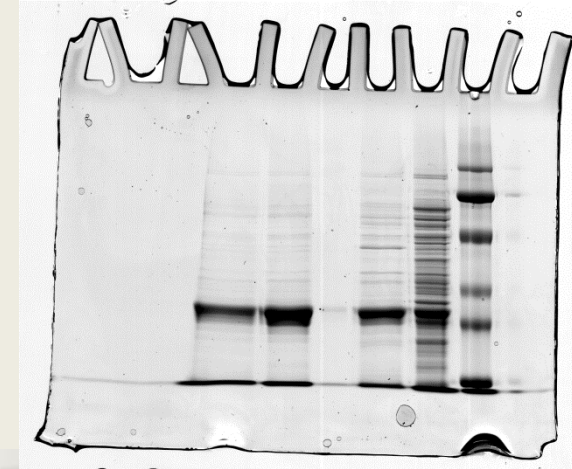
SDS PAGE – polyakrylamidová elektroforéza
