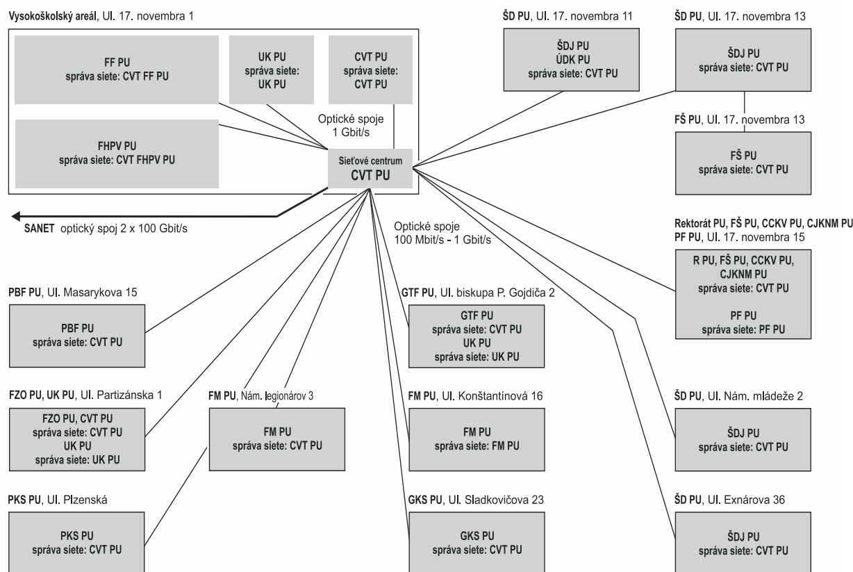
Obrázok 2: Schéma sieťového prepojenia objektov PU a správy sietí
