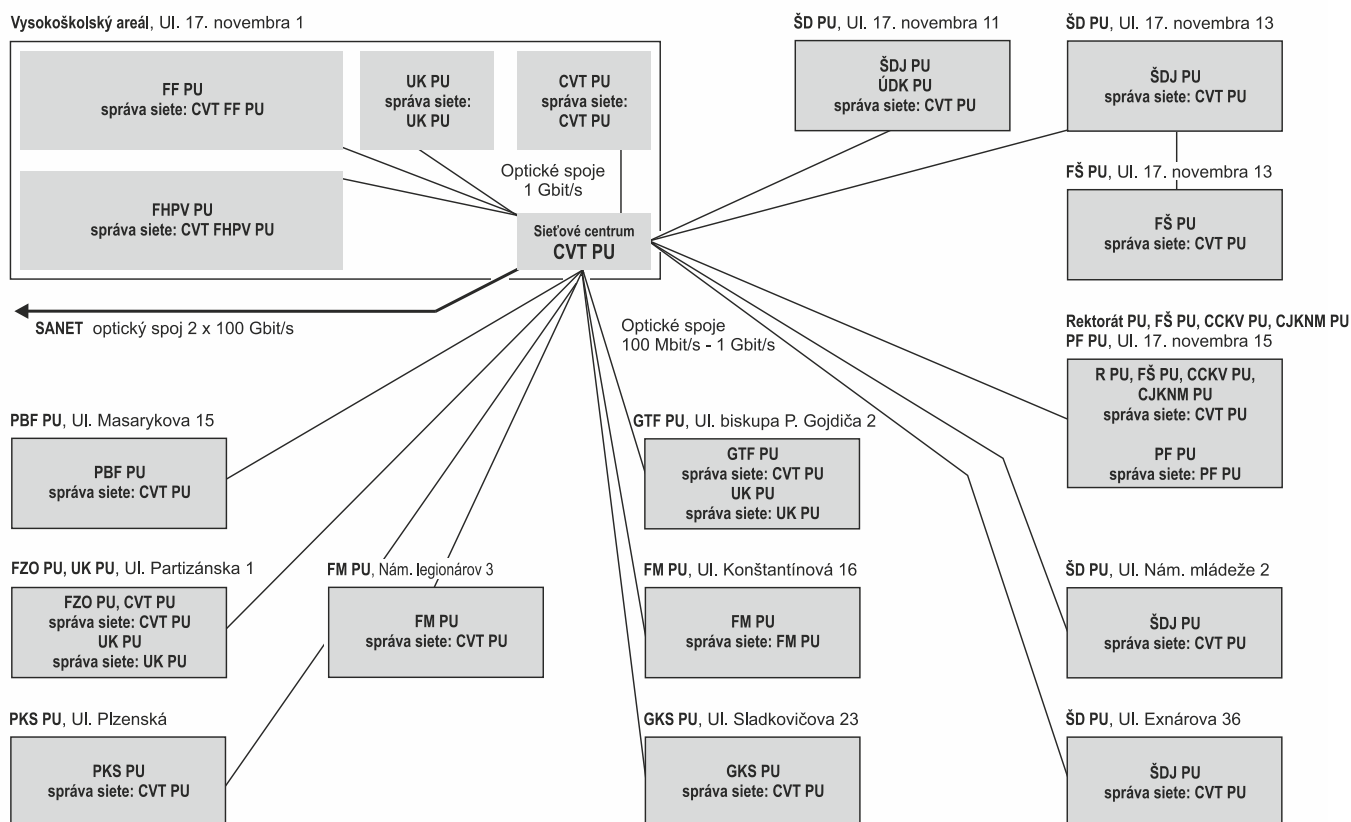
Obrázok 3: Schéma sieťového prepojenia objektov PU a správy sietí
