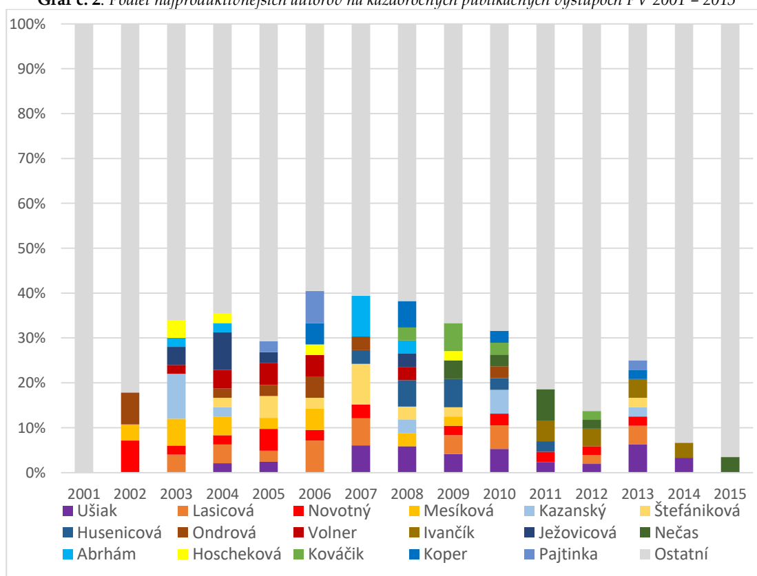
Graf č. 2: Podiel najproduktívnejších autorov na každoročných publikačných výstupoch PV 2001 – 2015
